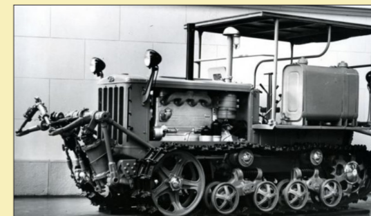
Гусеничный трактор
